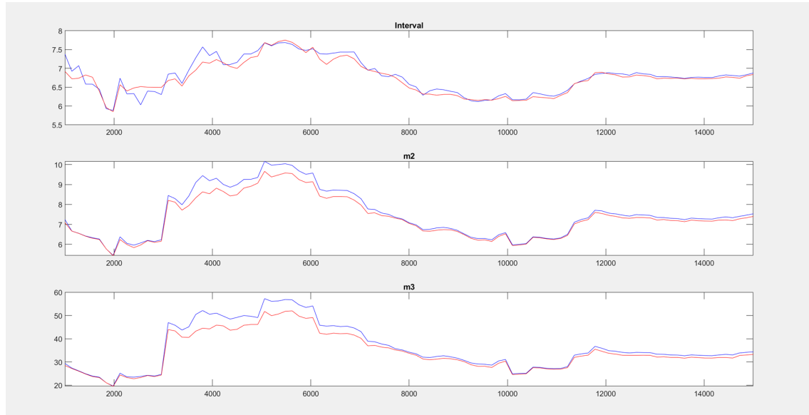
Figure 1: Test de convergence multivarié des paramètres du modèle - Brooks et Gelman, 1998
