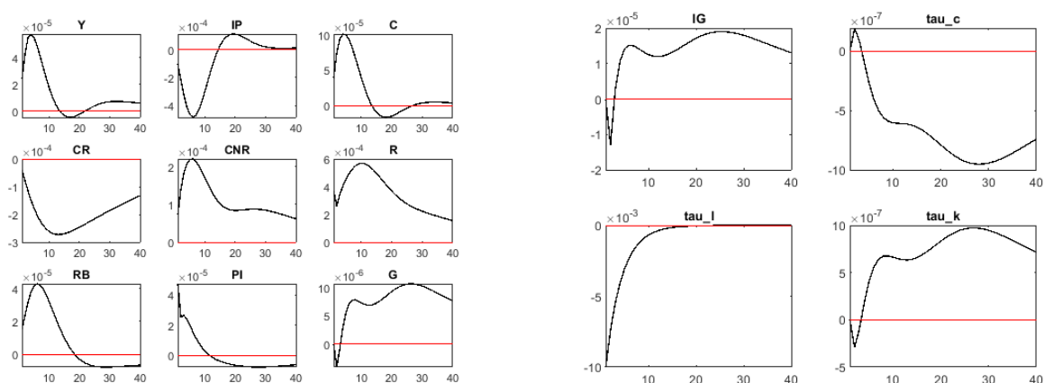
Figure 4: Orthogonalized shock to e_{\tau_l} : baisse de la taxe sur le revenu
