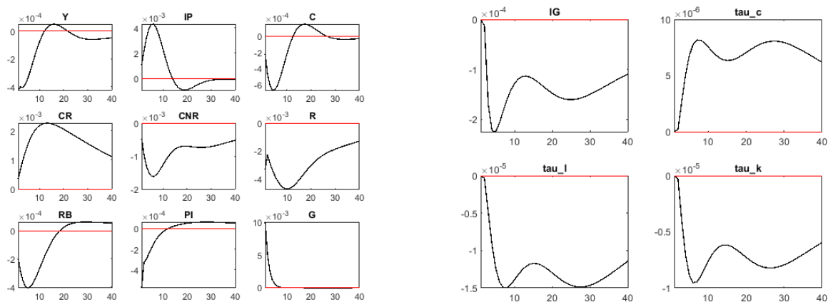
Figure 1: Orthogonalized shock to e_G : augmentation des dépenses publiques
