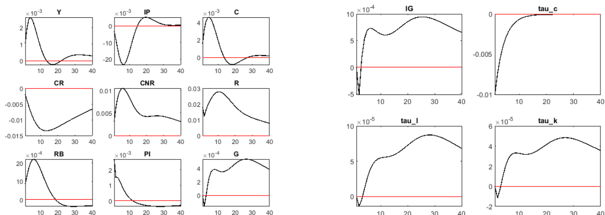
Figure 3: Orthogonalized shock to e_{\tau_c} : baisse de la taxe sur la consommation
