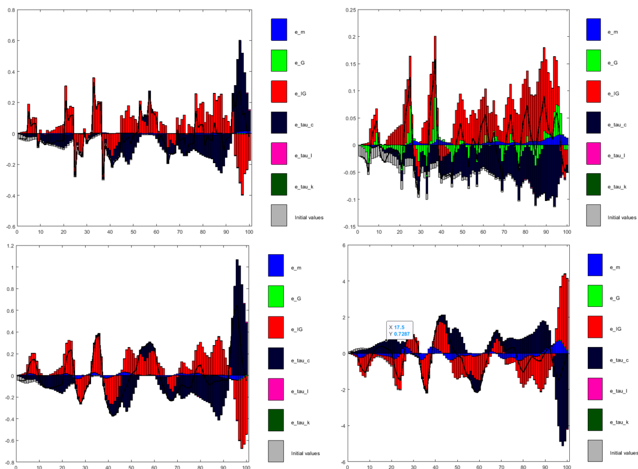
Figure 6: historical shock decomposition of Y, G, C and IP : de la gauche vers la droite
