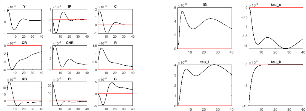
Figure 5: Orthogonalized shock to e_{\tau_k} : baisse des impôts sur le capital
